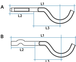
A Soportes para atornillar B Soportes para empotrar (obra)
