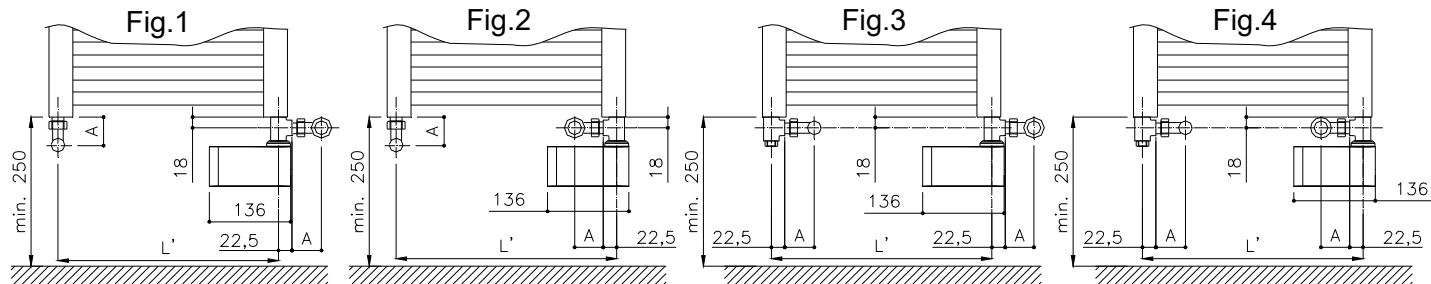
L' : entraxe hydraulique radiateur. A : dimension robinet equerre. Dimensions: (mm)
