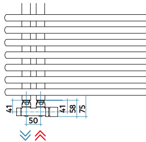
Tip s kolektorima na lijevoj strani Hidraulički priključak 50 mm
