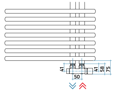
Tip s kolektorima na desnoj strani Hidraulički priključak 50 mm
