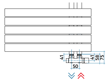
Instalare cu colectori în dreapta Conexiune hidraulică 50 mm
