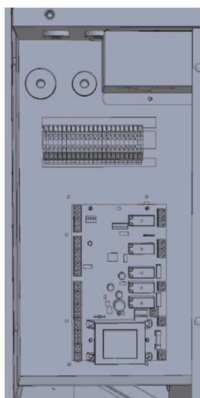
Quadro elettrico IRSAIR V 600
