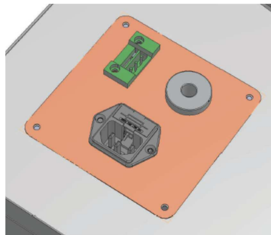
Collegamento elettrico pannello di comando E all'unità
