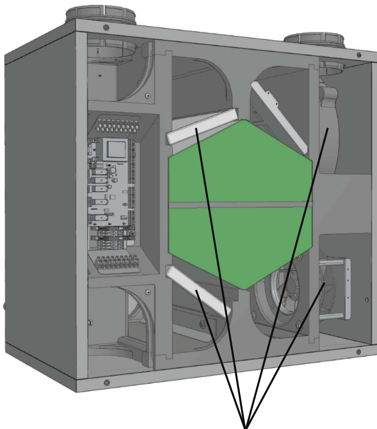
Filtr e ventilatori IRSAIR V 430 e 600
