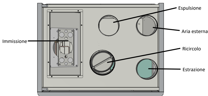
Collegamenti aeraulici – vista dall'alto
