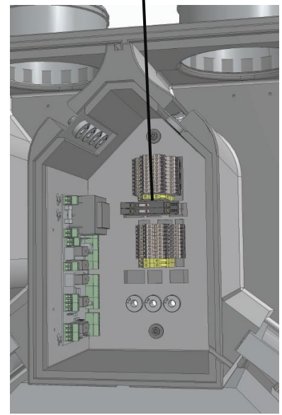
Fusibili e morsetteria elettronica tipo L
