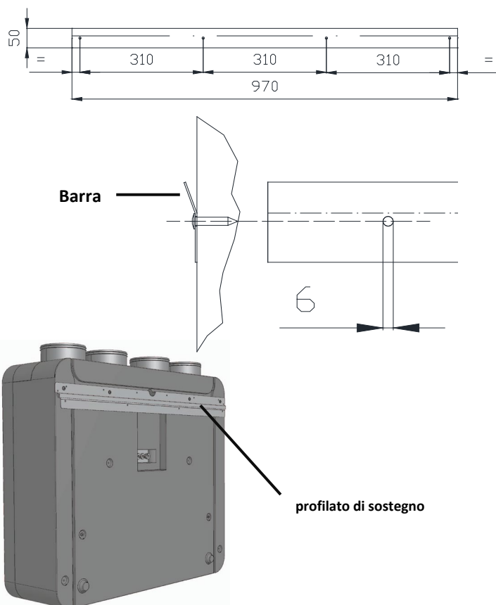
Montaggio a parete
