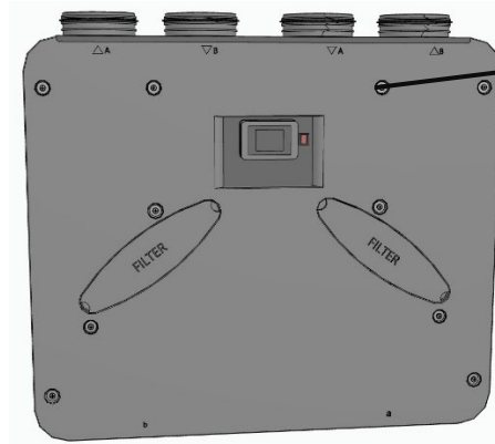
Fusibili e morsetteria elettronica tipo S
