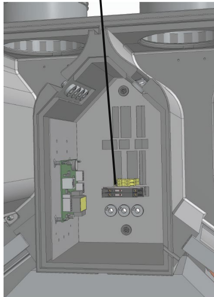
Fusibili e morsetteria elettronica tipo S
