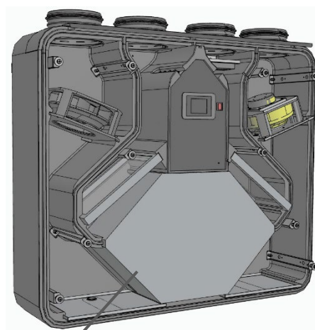
Scambiatore di calore
